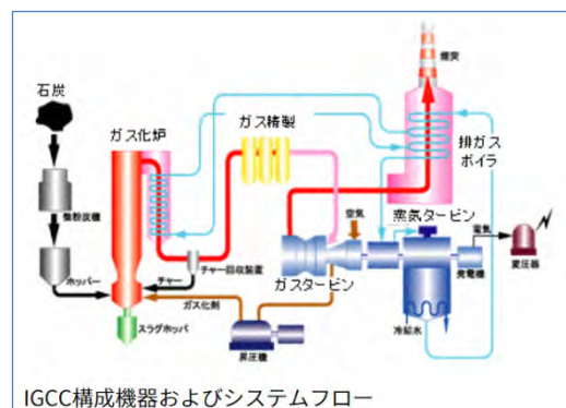
IGCC構成機器およびシステムフロー
