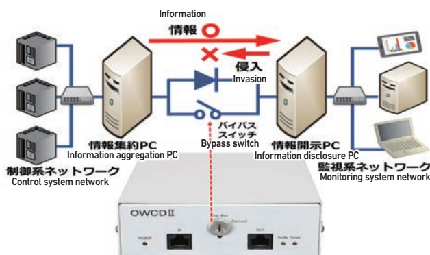
通信セキュリティ装置 OWCD (One Way Control Device)
