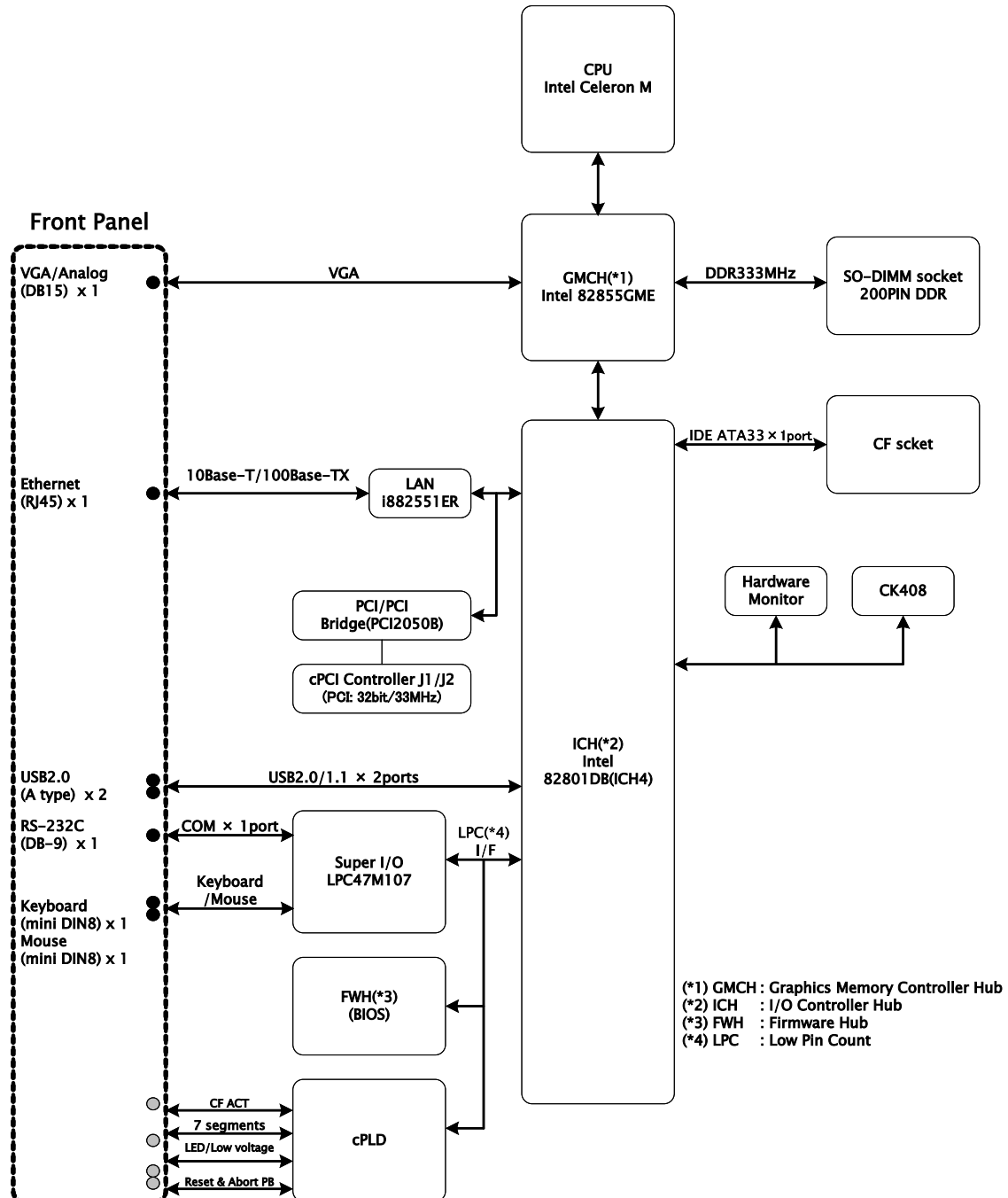
CPCPU31 ブロック図
